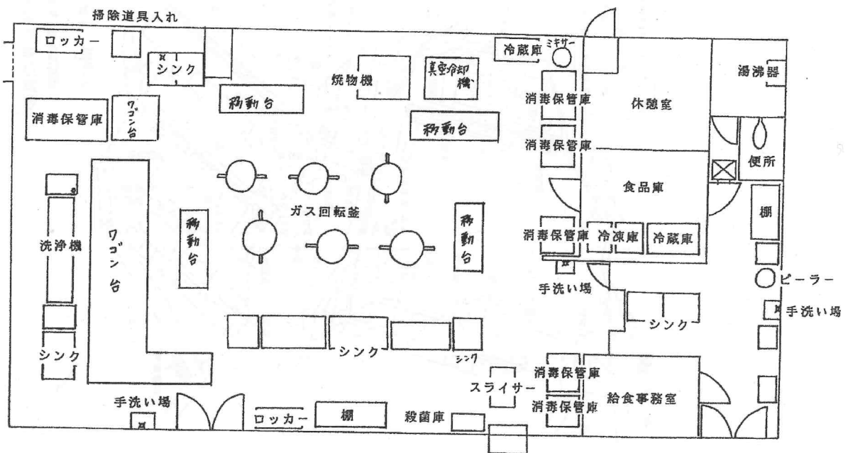
給食室 平面図 1/100
